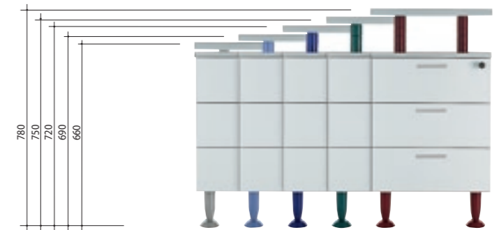
Regolazione cassettiera portante. Adjusting the carrying pedestal. Réglage du caisson porteur. Einstellung des tragenden Schubladenelements. Regulación cajonera portante. Regulagem do gaveteiro pedestal.
