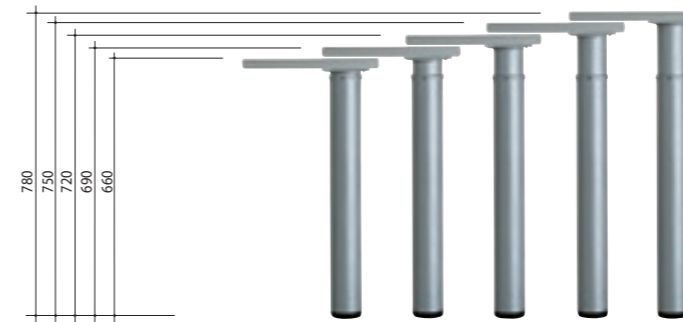
Regolazione gamba metallica. Adjusting the metal leg. Réglage du pied métallique. Einstellung des Metallbeins. Regulación pata metálica. Regulagem do pé metálica.
